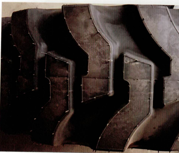
Pneu 17,5 R 25
